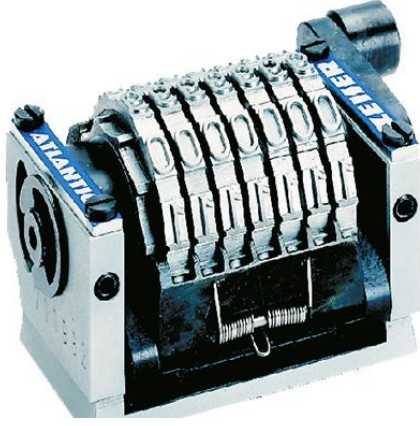
Şekil.1 Model 300 Numaratör
