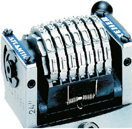
Şekil.2 Model 200 Numaratör
