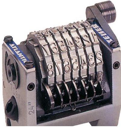
Şekil.1 Model 100 Numaratör
